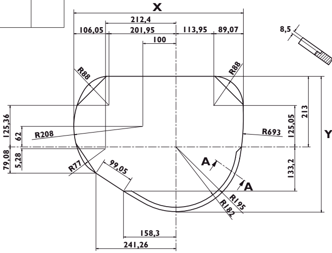
SEZ. A-A
